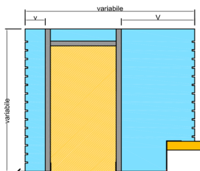
Cassonetto "MBF" per frangisole maggiorato
