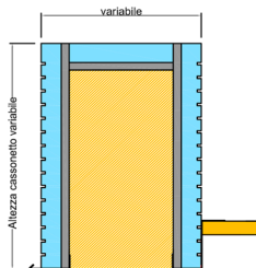
Cassonetto "MBF" per frangisole
