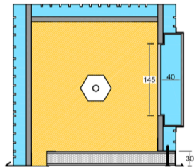
Cassonetto "MBI" ispezione frontale
