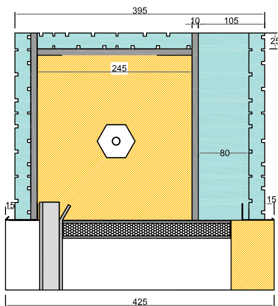
Cassonetto MB 395 con cielino Brandeggiante Parete maggiorata da 80 mm trasmissione termica U_{sb}=0,36 \text{ W}/(\text{m}\cdot\text{K})
