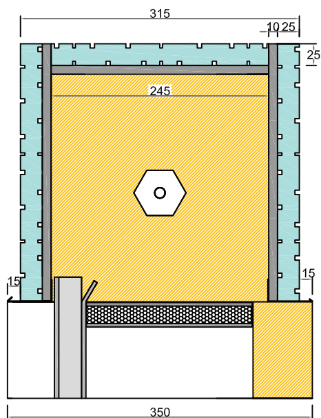
Cassonetto MB 315 standard
