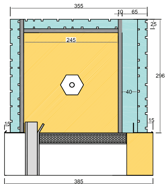
Cassonetto MB 355 con cielino Brandeggiante Parete maggiorata da 40 mm trasmissione termica U_{sb}=0,49 \text{ W}/(\text{m}\cdot\text{K})
