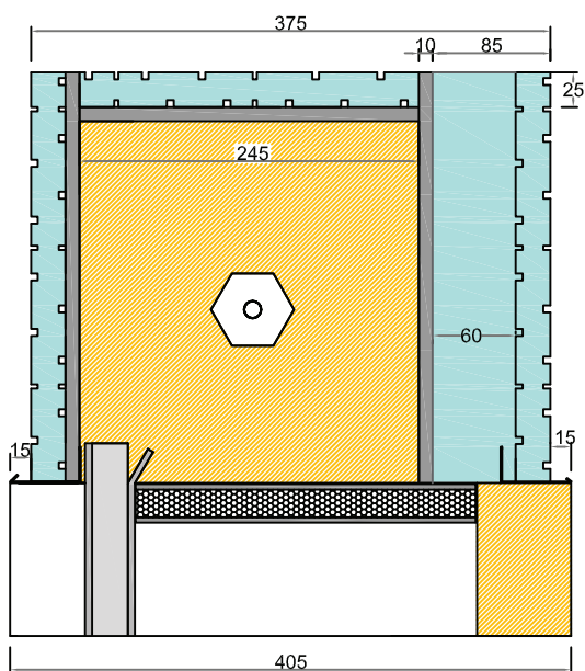
Cassonetto MB 375 con cielino Brandeggiante Parete maggiorata da 60 mm trasmissione termica U_{sb}=0,41 \text{ W}/(\text{m}\cdot\text{K})
